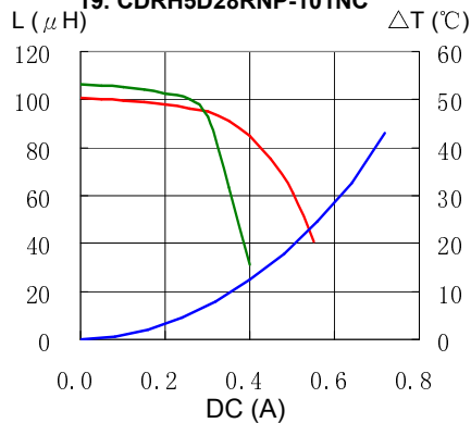
19. CDRH5D28RNP-101NC
