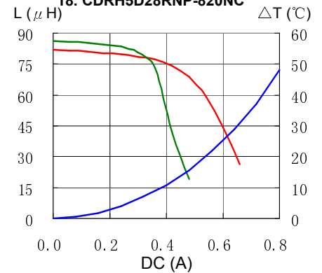
18. CDRH5D28RNP-820NC
